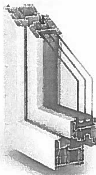
Nárez plastové okno TROCAL 88+
